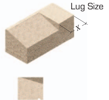
LUG END
